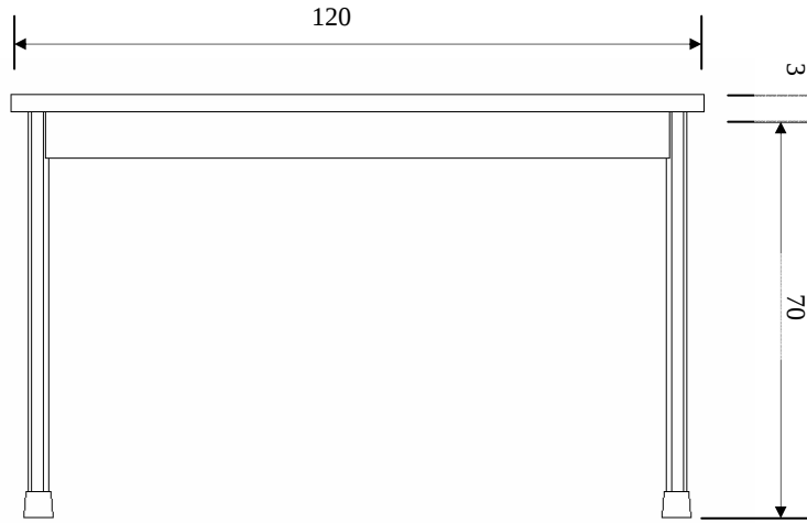
ÖN GÖRÜNÜŞ
