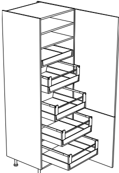
5 Teleskobik İç Çekmece, 2 Kapak, 1 Sabit Raf, 1 Seyyar Raf, *Modül yönü; Sağ (R)
