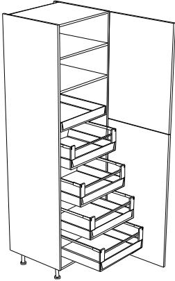
5 Teleskopik İç Çekmece, 2 Kapak, 1 Sabit Raf, 1 Seyyar Raf,
