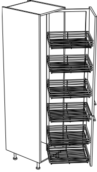
Starax sistemi, 6 Rafli tel sepet,
