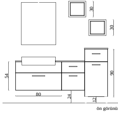
ön görünüş
