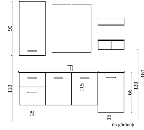
ön görünüş
